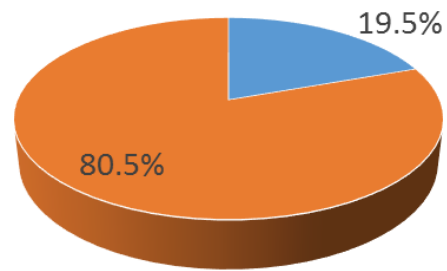
Carbon Budget 2011-2050 World - 1386.6 GtCO 2 eq
